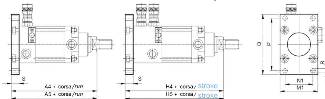
Flangia posteriore in alluminio
