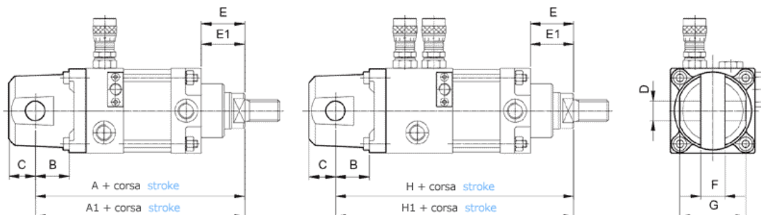
Cerniera posteriore in alluminio
